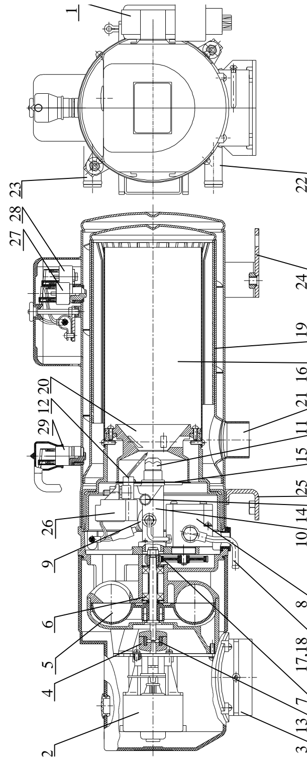
Рисунок 1 - Подогреватели 15.8106-03 и 151.8106-03:
