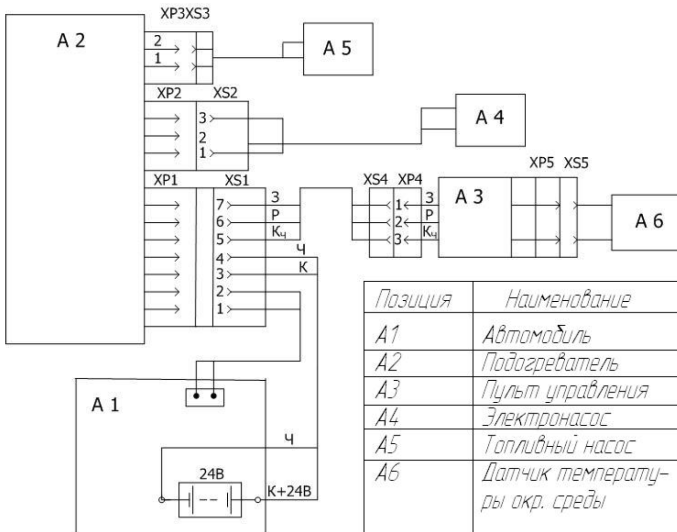
Рис.1 Схема электрических соединений подогревателя «ПРАМТРОНИК 18Д-24»
