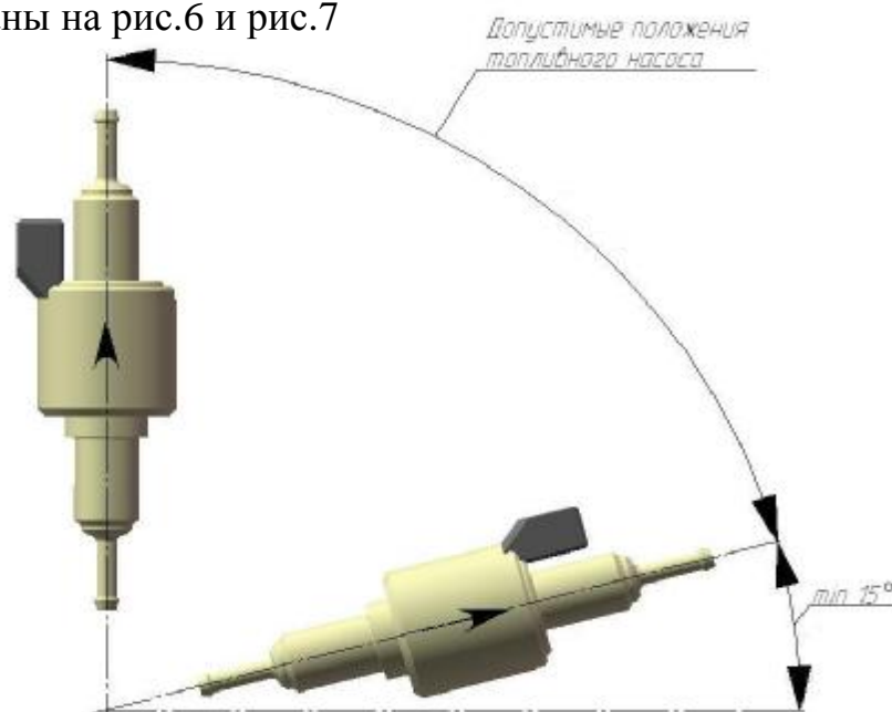
Рис. 5 Допустимые монтажные положения топливного насоса
