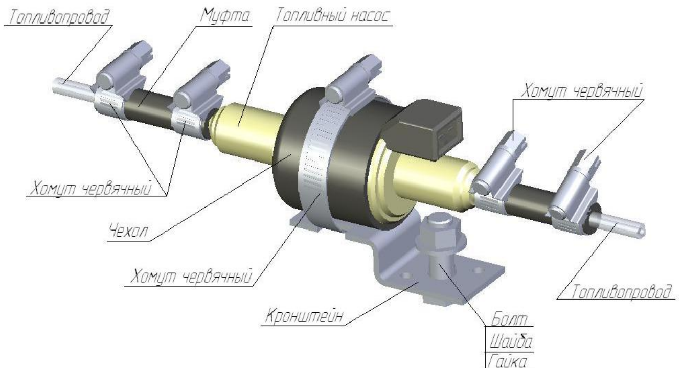
Рис. 9 Схема монтажа топливного насоса
